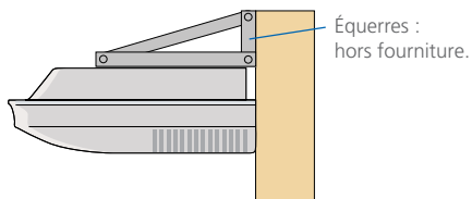
Installation au mur
